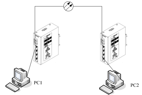
图 4-2 光口测试
