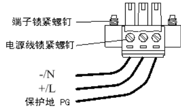
图 3-5 直流电源端子接线图
