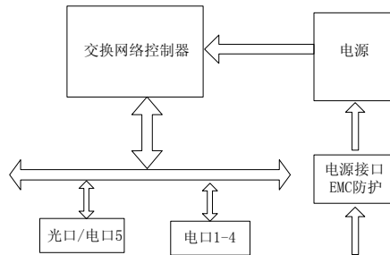
图 3-1 硬件结构
