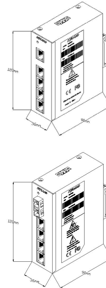
图 3-2 产品外形图
